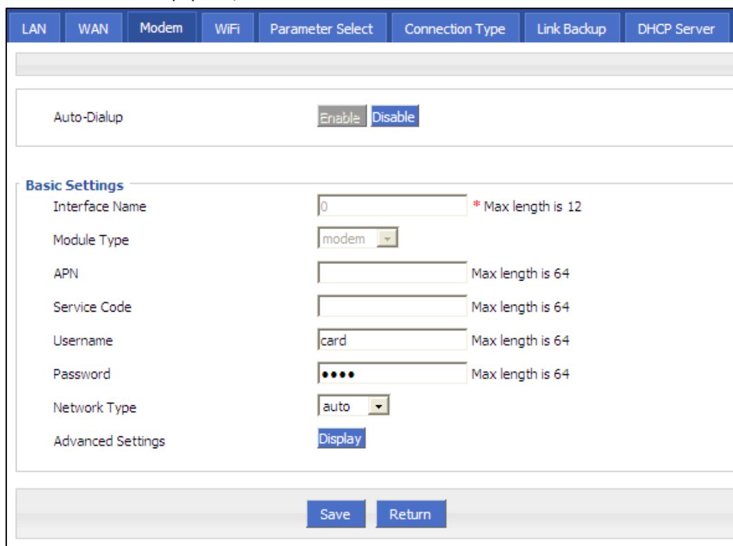
Рис. 3.3.2.3-2: Подключение к сотовой сети
