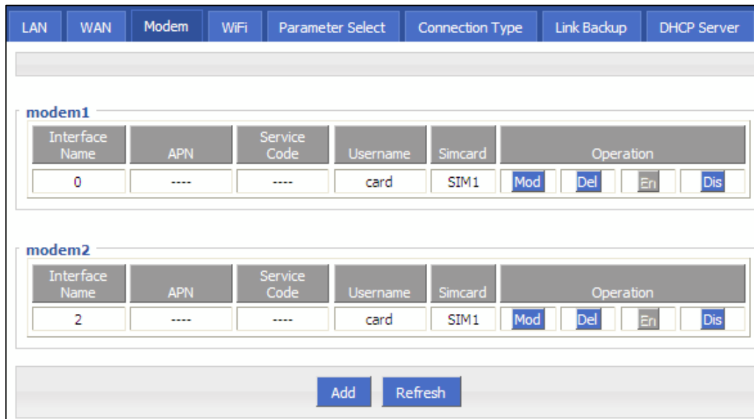
Рис. 3.3.2.3-1 Модем (modem)
