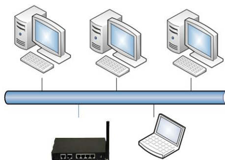
Рис. 3.2.2.2: Метод подключения 2
