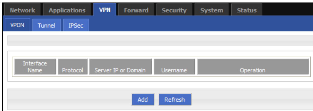
Рис. 3.3.4 VPN
