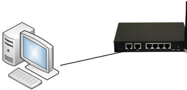
Рис. 3.2.2.1: Метод подключения 1
