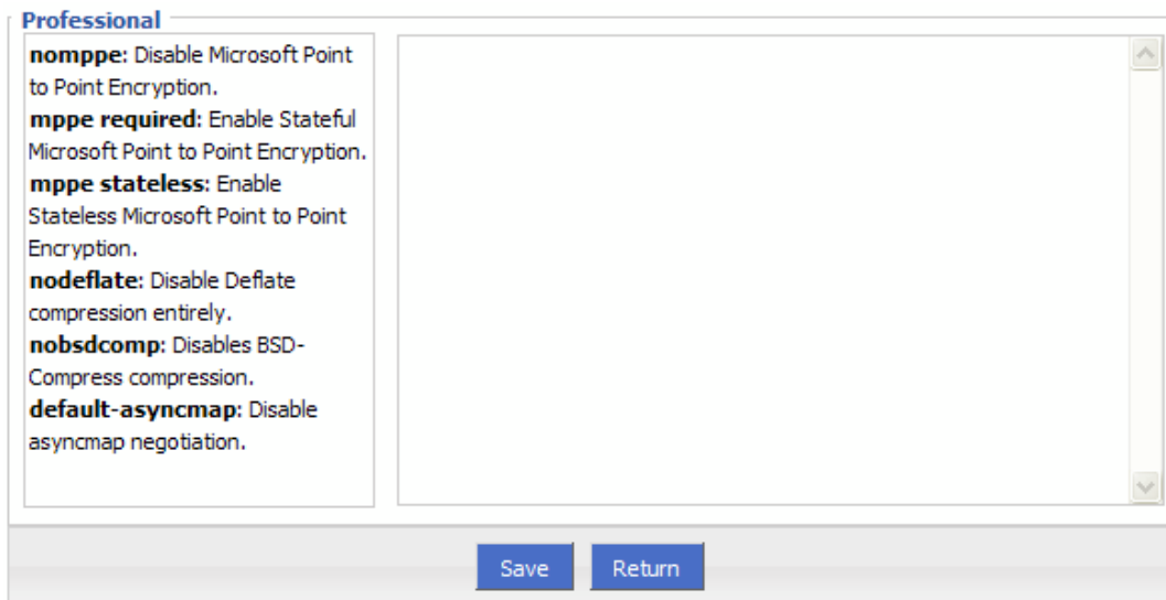
Рис. 3.3.2.2-3: Дополнительные настройки
