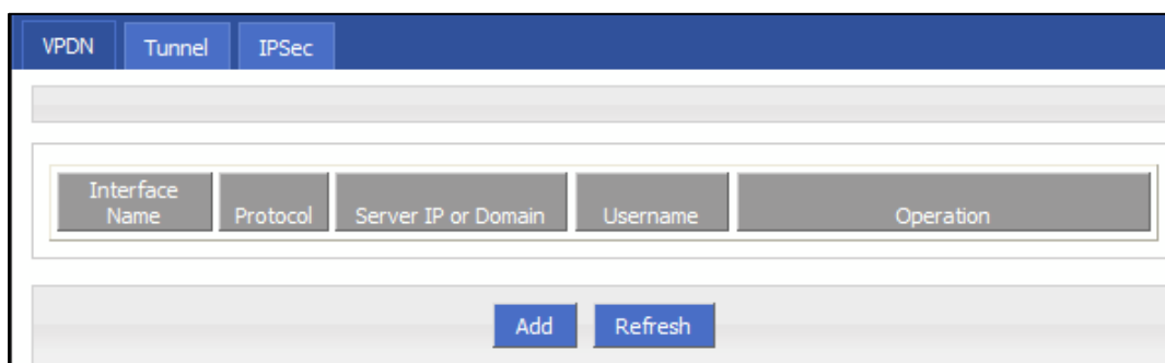
Рис. 3.3.4.1 VPDN
