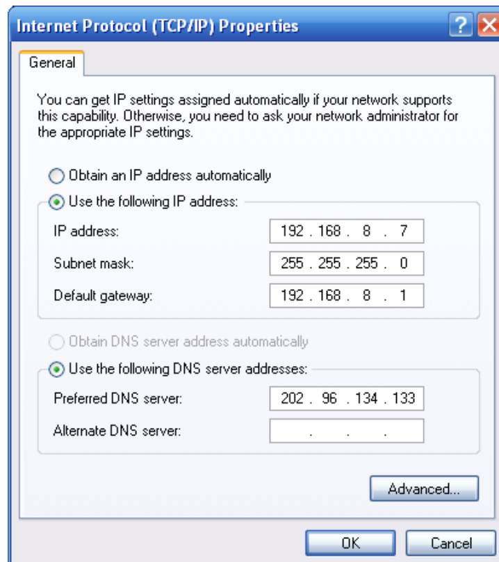
Рис. 3.2.3-3: TCP/IP-свойства
