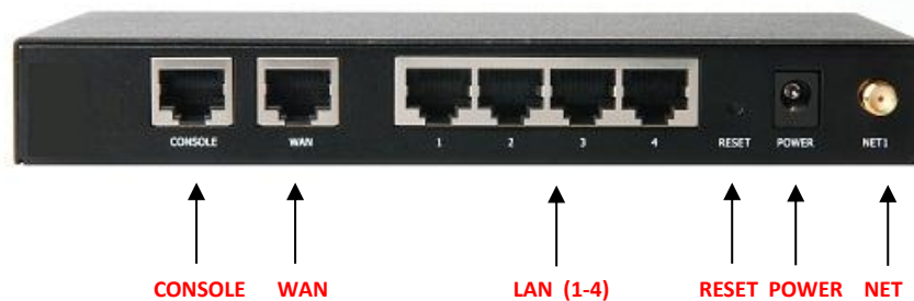
Рис. 2.1.1-2: Задняя панель (модель без встроенного Wi-fi-модуля 2 )
